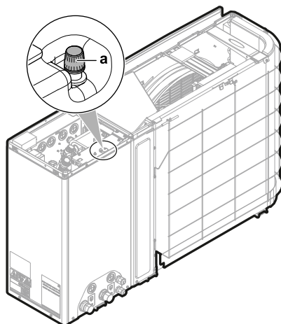
a Schräder-Ventil
