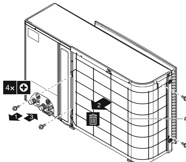
a Ansaugluftgitter
